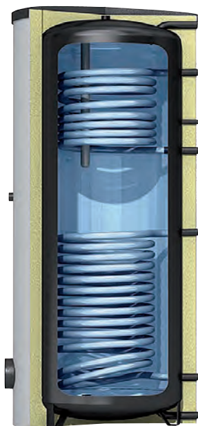
Modello RS-2 con due scambiatori di calore integrati a tubo liscio
